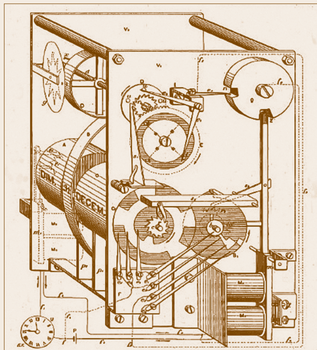
Kleiszner villamos óranaptárának rajza a párizsi La Lumière Électrique 1889. március 2-i számában
